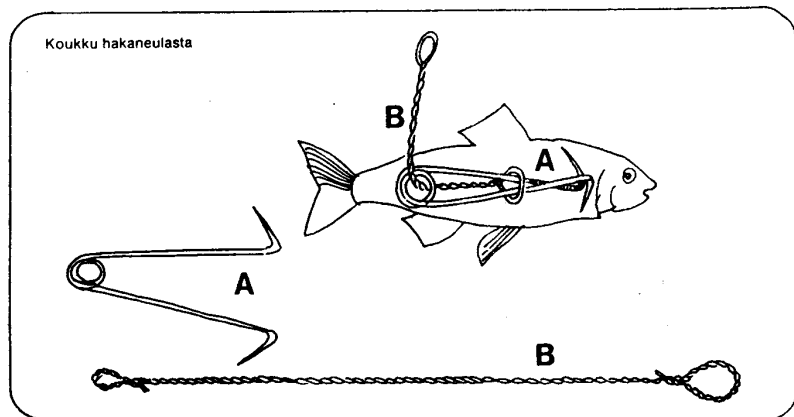
Kuva 7. Koukkupyynti talvella.
